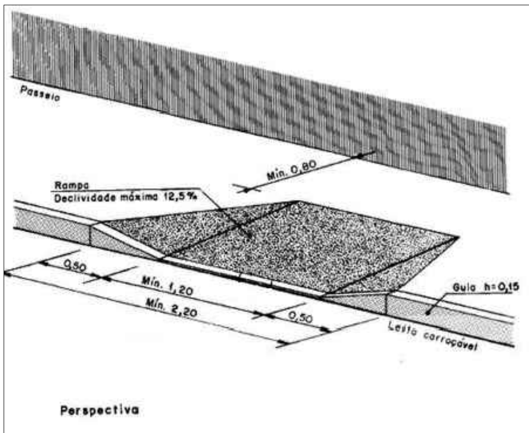
DETALHE REBAIXO DA CALÇADA PARA PEDESTRES-RAMPA DE ACESSO PARA CADEIRANTES S/ ESCALA
